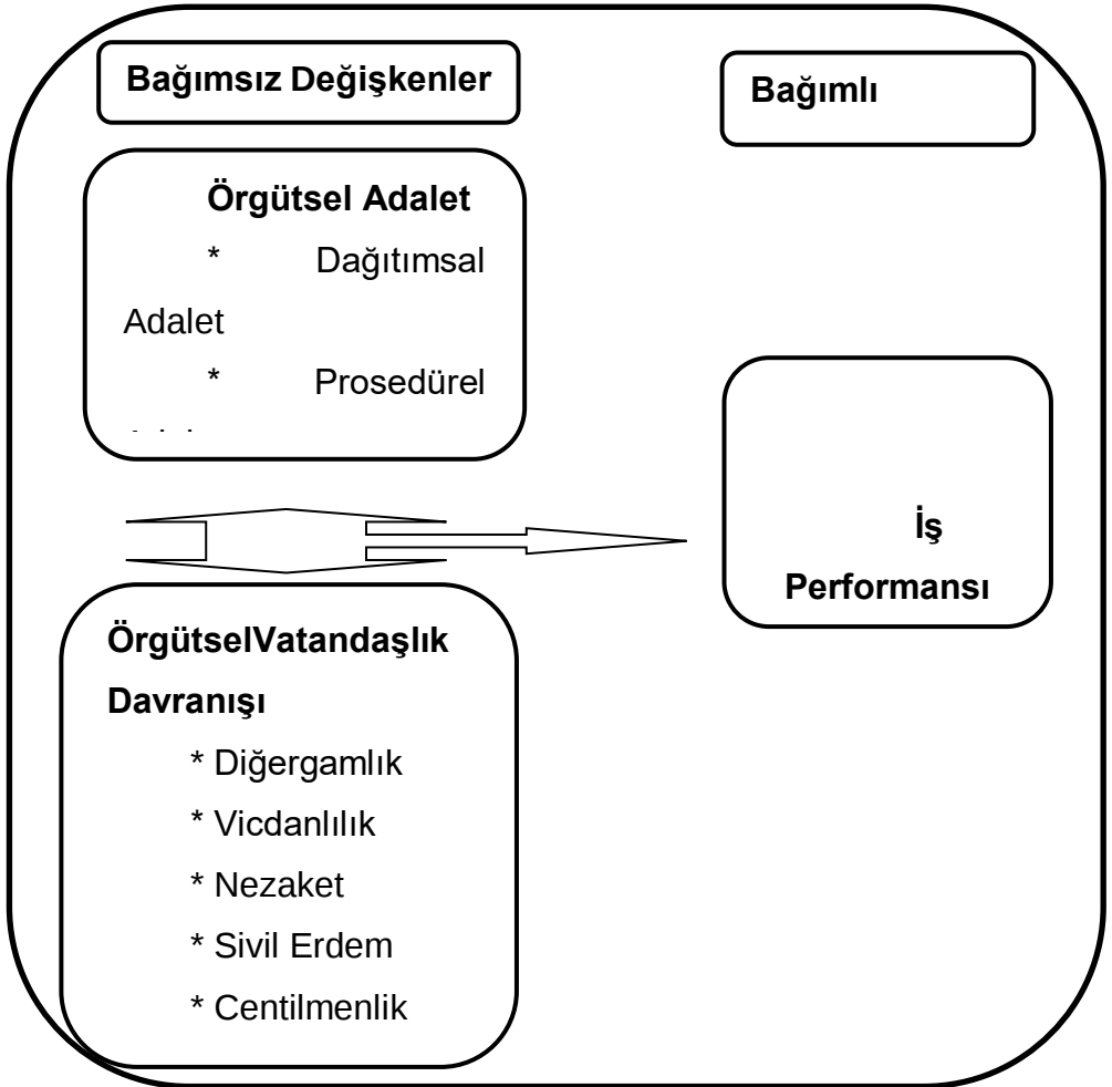
Şekil 2 Araştırmanın Modeli
